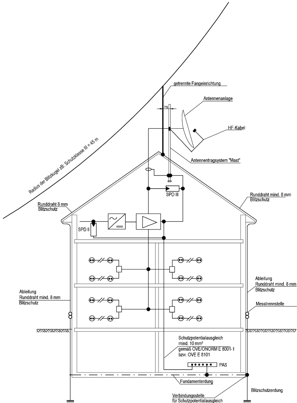
Bild 1 – Beispielhaftes Prinzipschaltbild für eine Antennenanlage im Schutzbereich einer Fangstange inkl. Überspannungsschutz und Schutzpotentialausgleich
