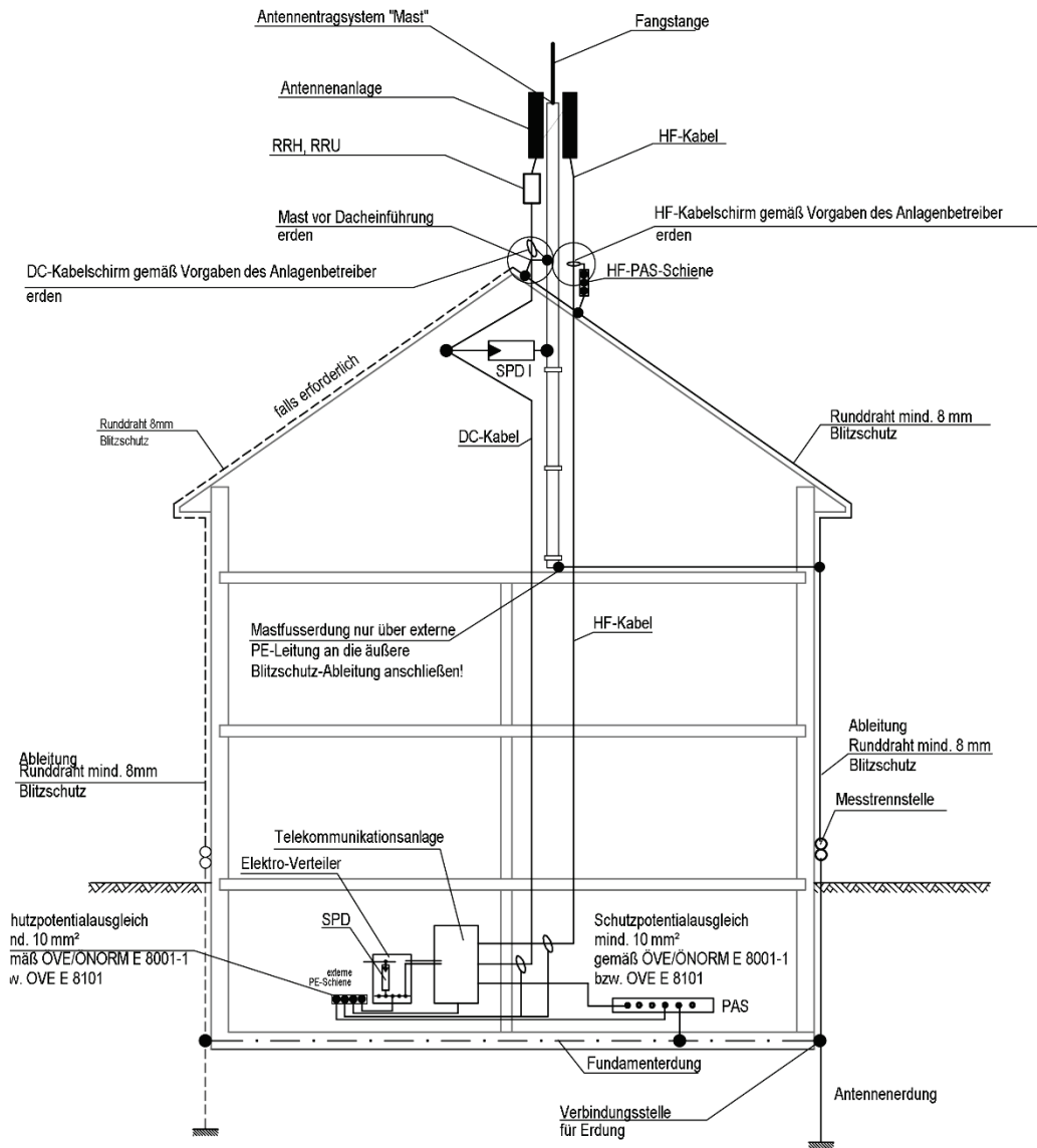
Bild 3 – Antennenanlage mit Blitzschutzsystem
