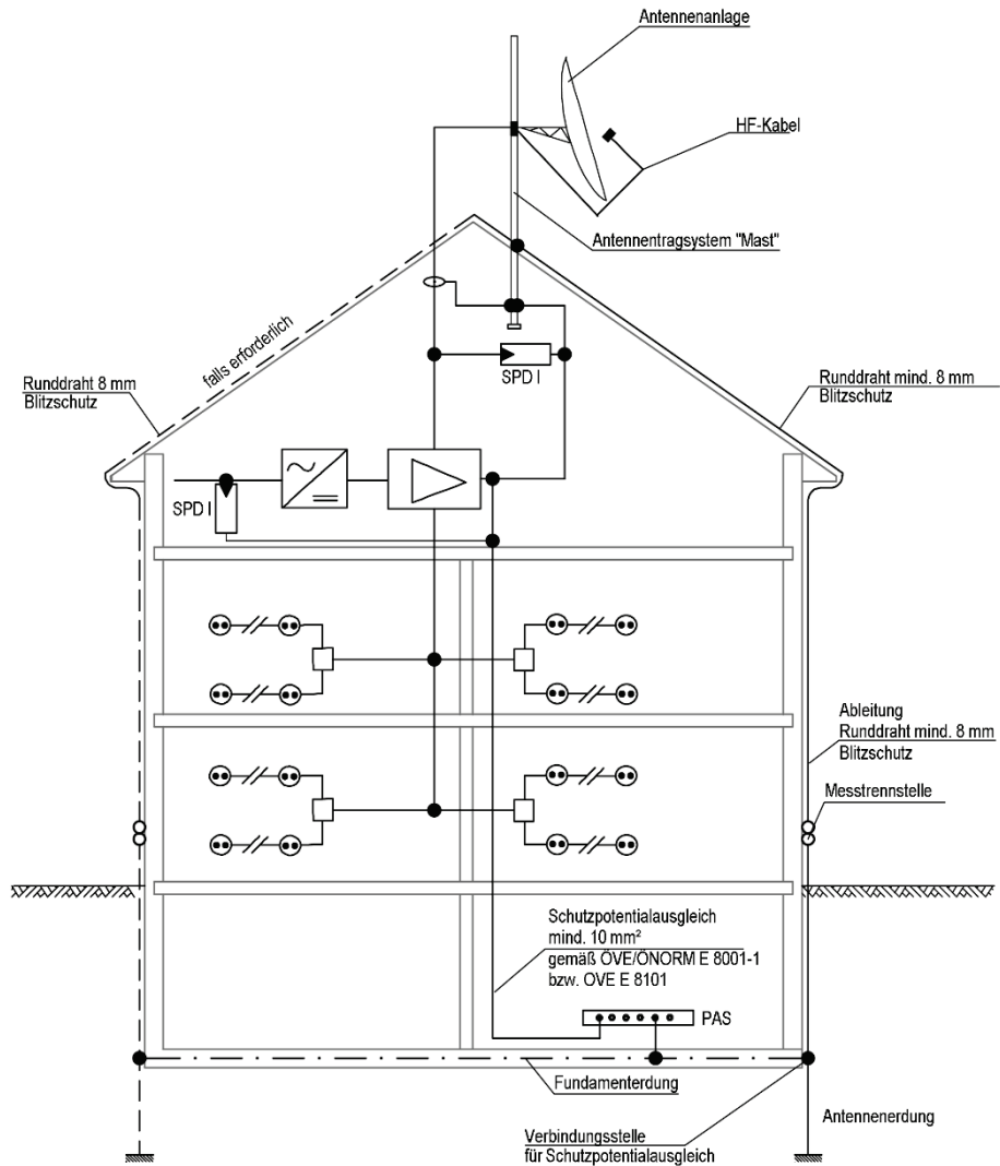
Bild 2 – Beispielhaftes Prinzipschaltbild für eine Antennenanlage, die direkt an die Erdleitung angeschlossen ist, mit einem Überspannungsschutz und Schutzpotentialausgleich
