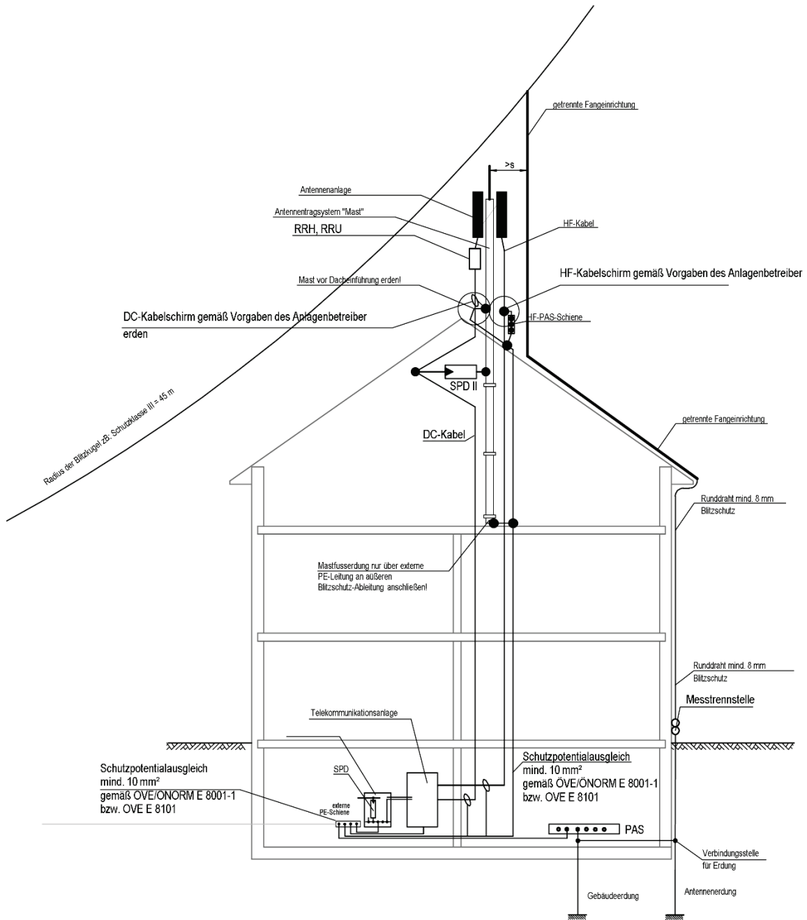
Bild 4 – Antennenanlage ohne Blitzschutzsystem
